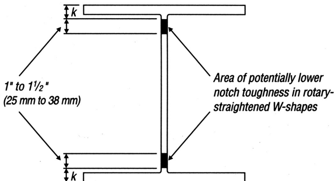
Fig. C-A3.1. "k-area."
